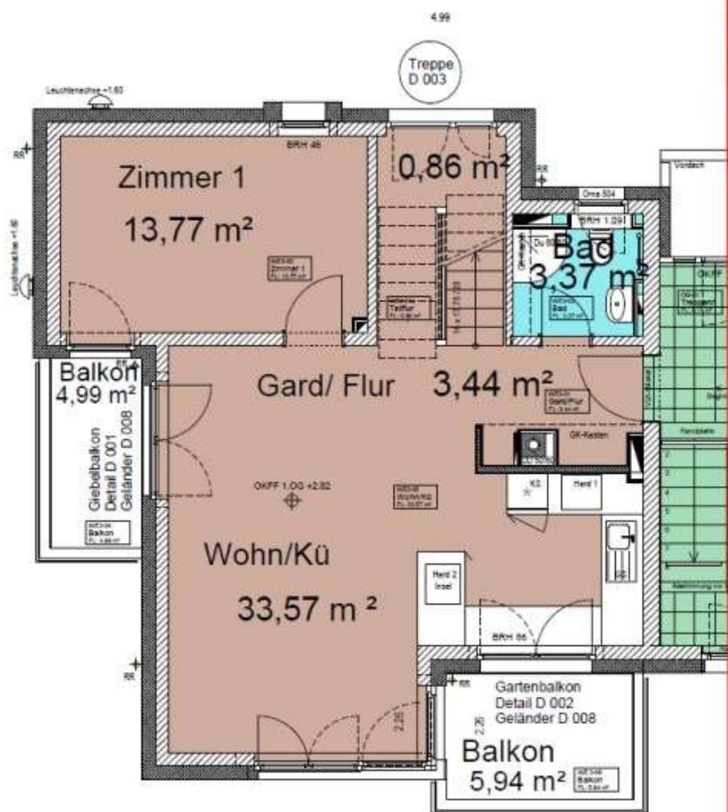
Grundriss 1. Obergeschoss - 1:50
